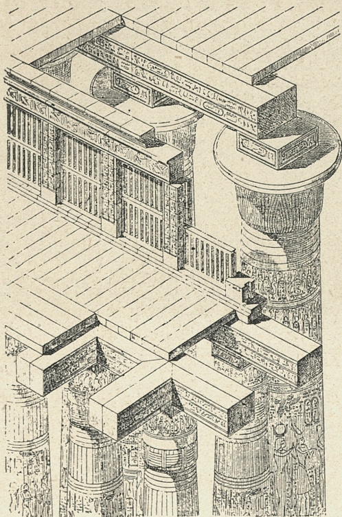
Fig. 14. — Éclairage par claire-voie dans la salle hypostyle du temple de Khons à Karnak. (D'après Perrot et Chipiez.)
