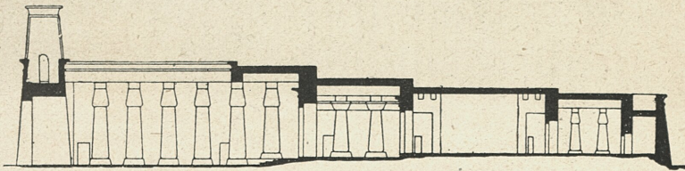
Fig. 12. — Diminution progressive de la hauteur des salles. Temple de Khonsou, à Thèbes.
