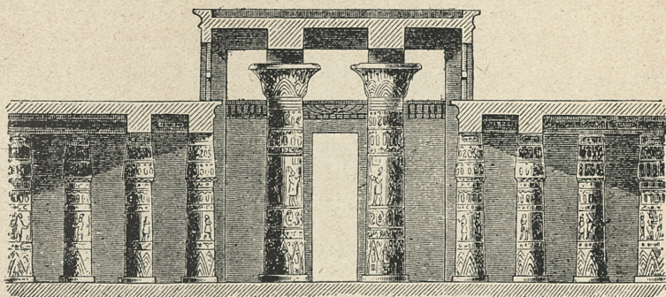
Surélévation de la double rangée de colonnes du milieu pour l'éclairage de la salle hypostyle du temple de Khons à Karnak.
