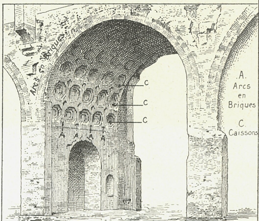
VOÛTE EN BERCEAU CONSTRUITE EN BLOCAGE ROME Basilique de CONSTANTIN
