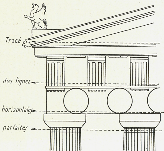
Fig. 2. — Convexité de l'entablement.
