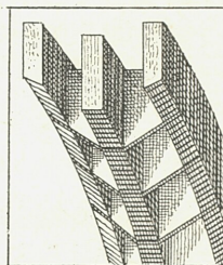
ARC DE VOÛTE D'ARÊTES EN BRIQUES
