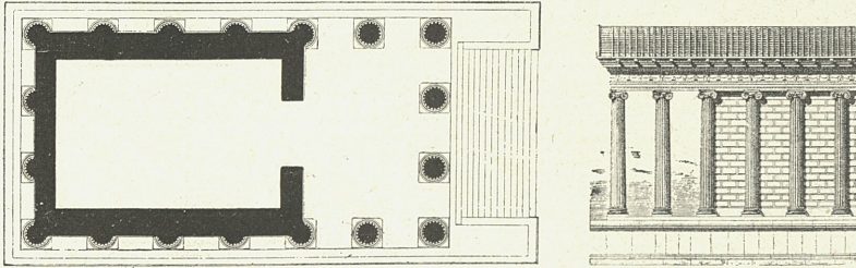
Fig. 21 et 22. — Plan et façade latérale du Temple de la Fortune virile, à Rome.
